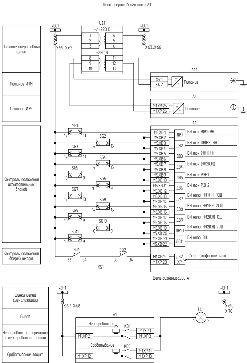
Рисунок В.2 – Схема электрическая принципиальная (часть 2)
